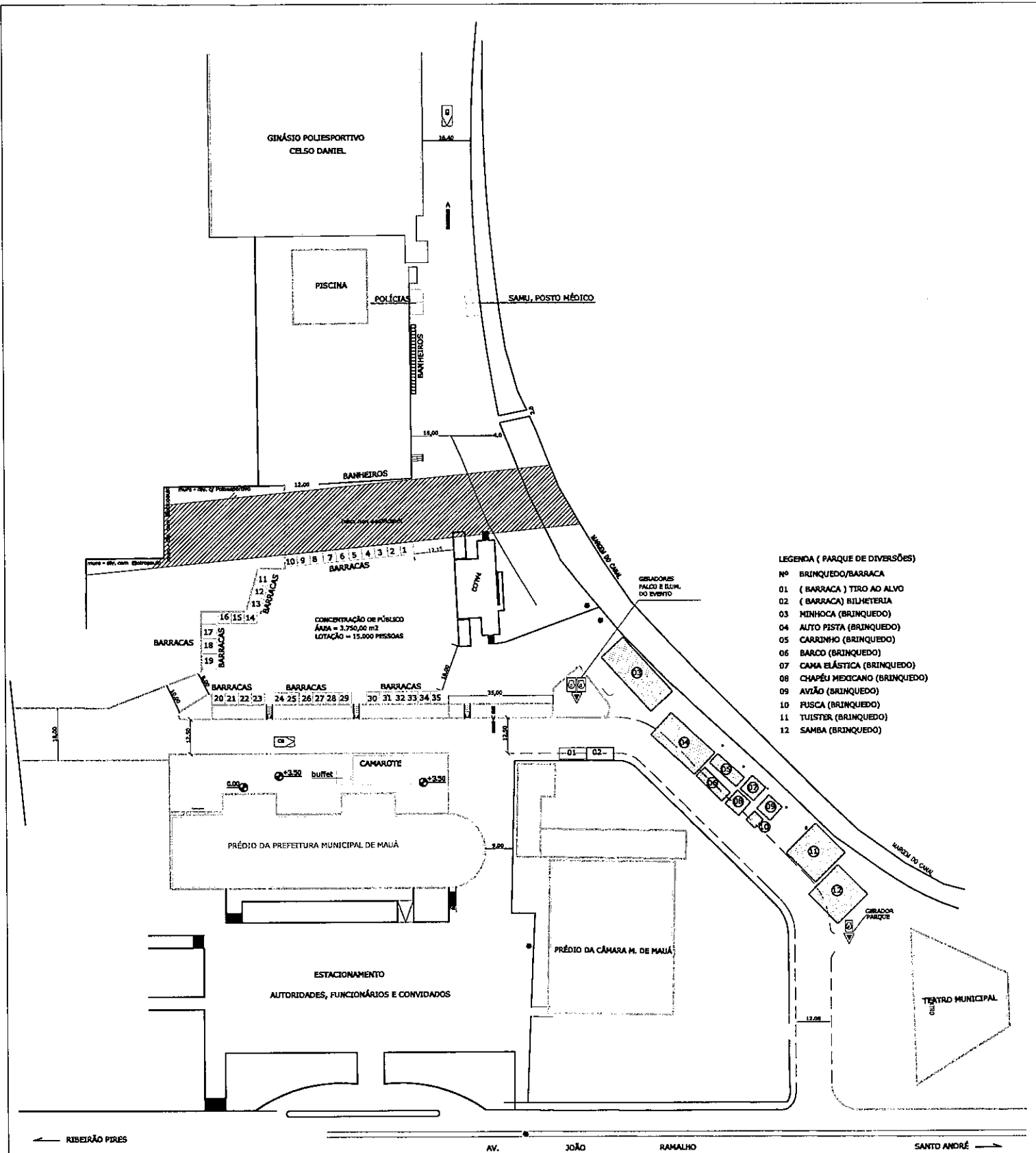
PLANTA BAIXA ESCALA 1:750
