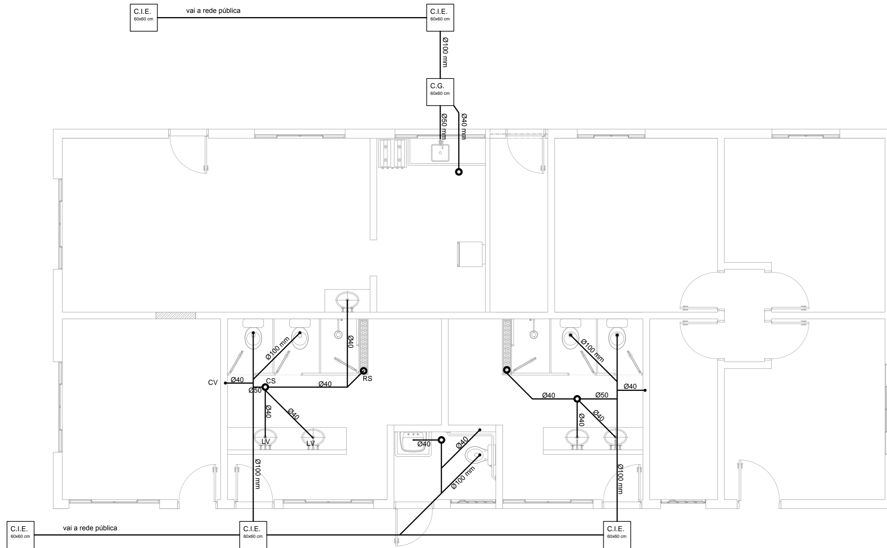
4 PLANTA - ESGOTO Sc1: 1:50
