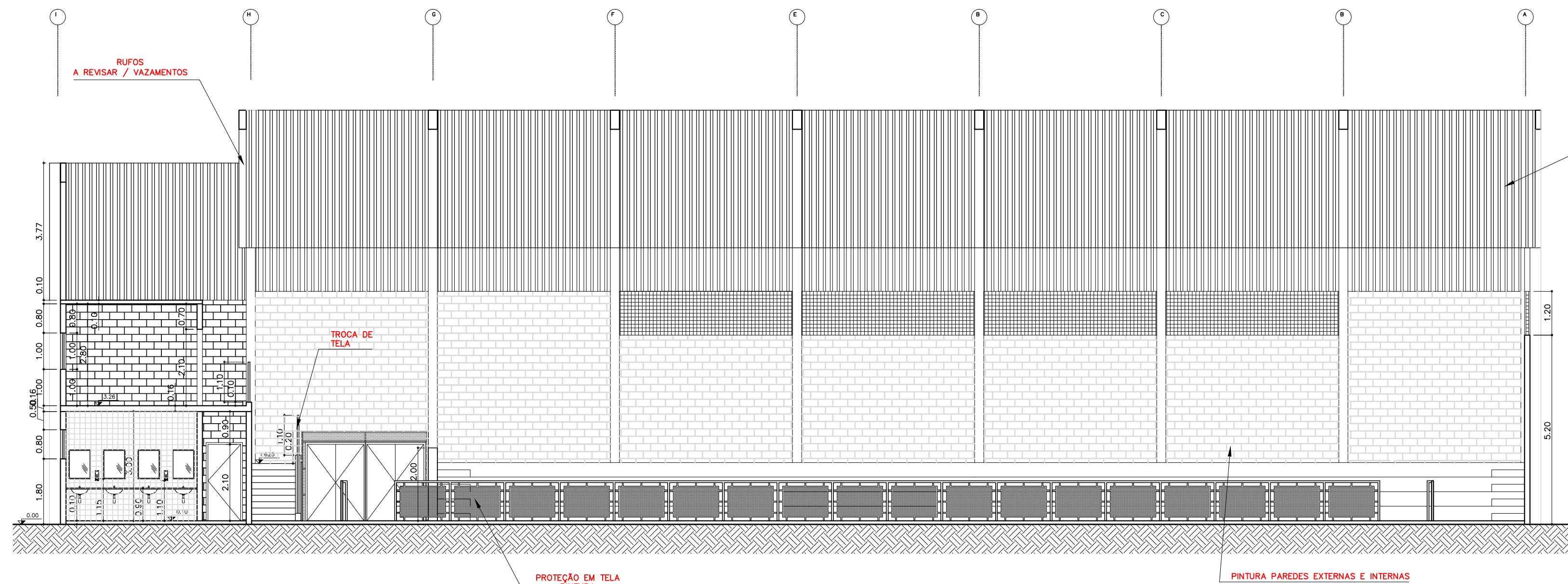
CORTE LONGITUDINAL
