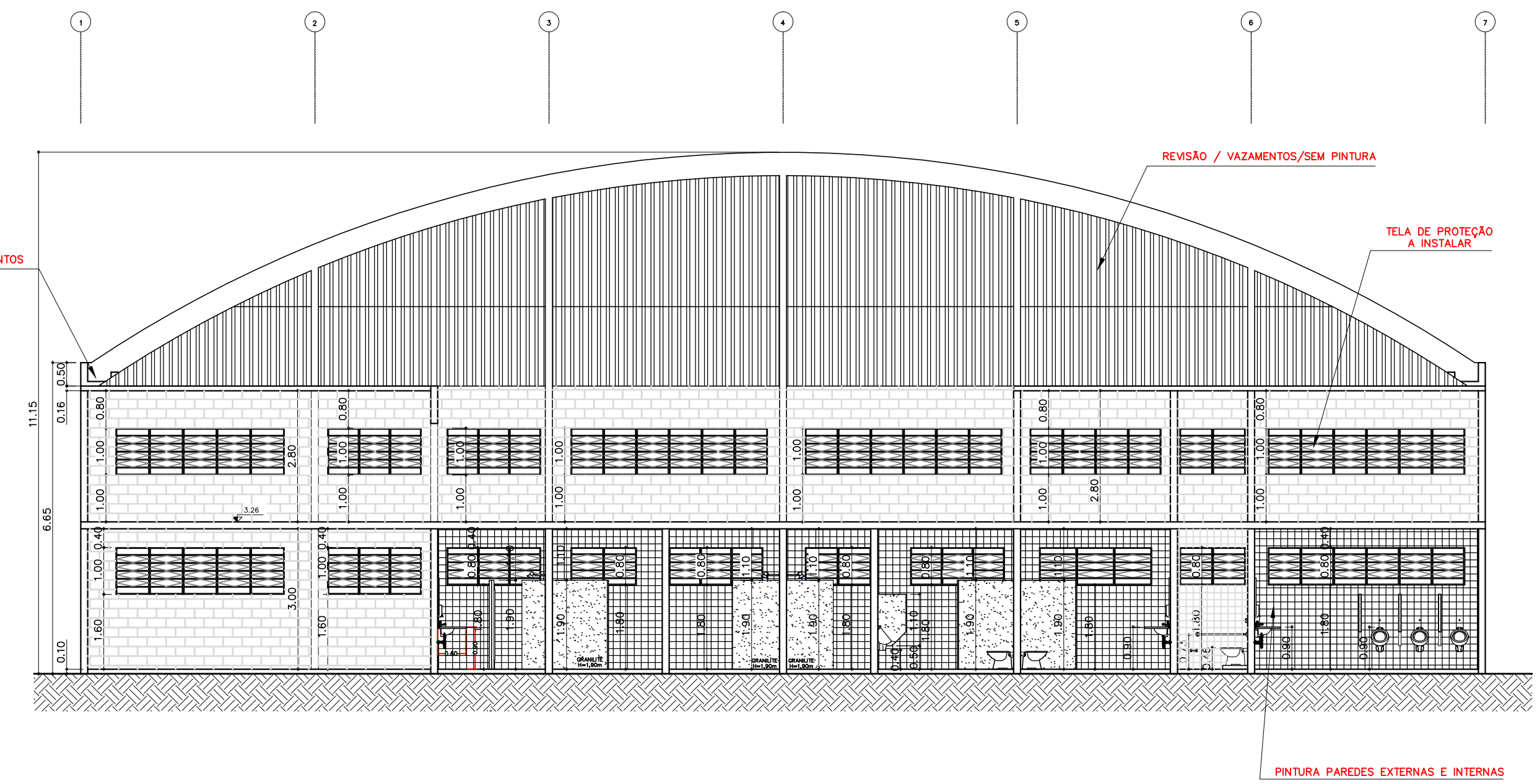
CORTE TRANSVERSAL
