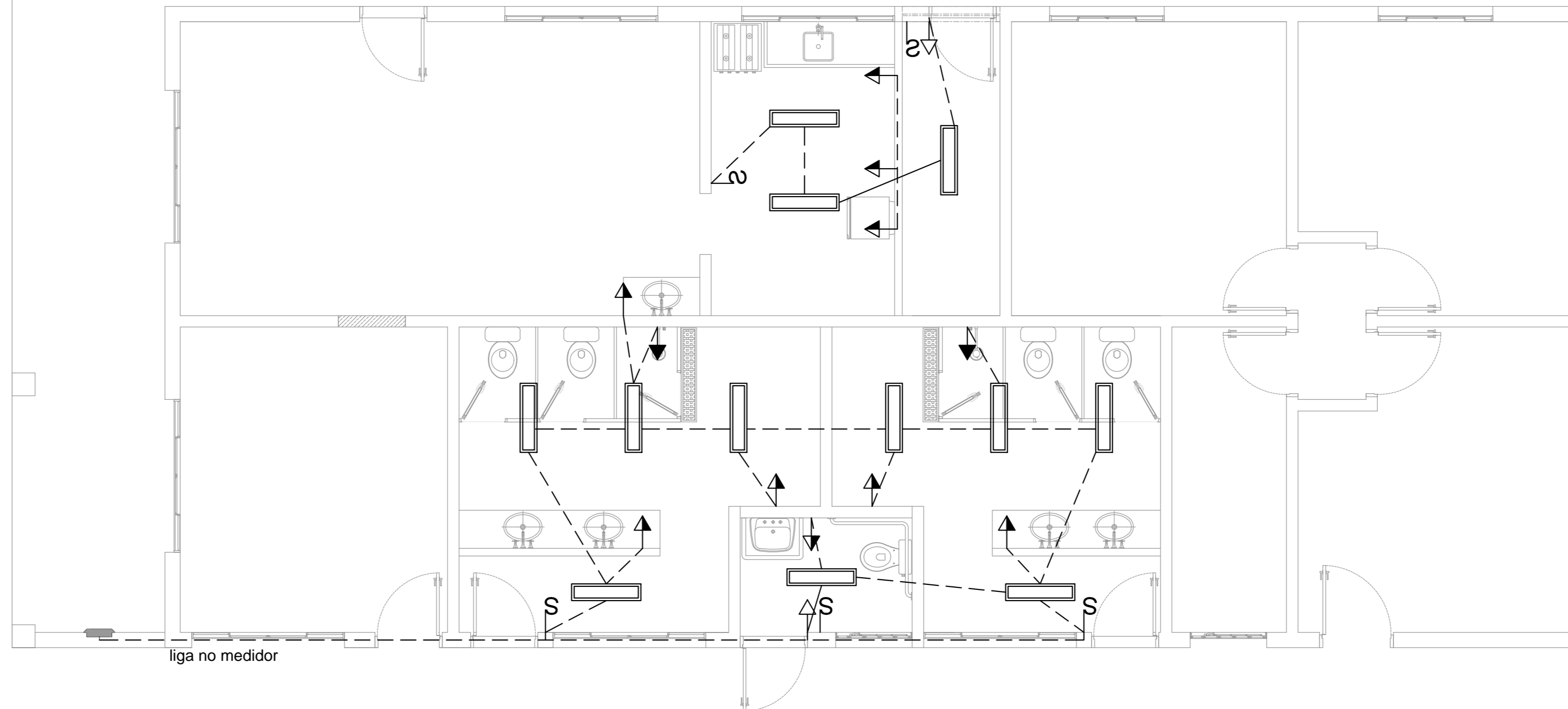
5 PLANTA - PONTOS DE ELÉTRICA Sc1: 1:50
