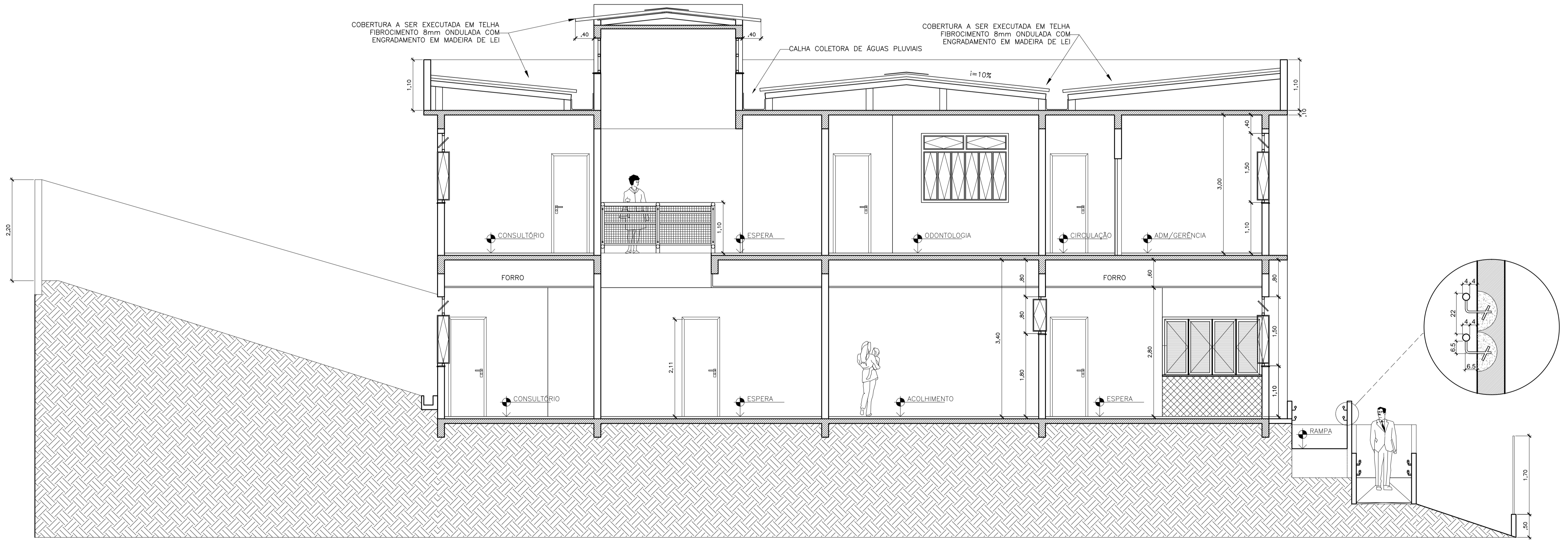
CORTE 2 ESCALA: 1:50
