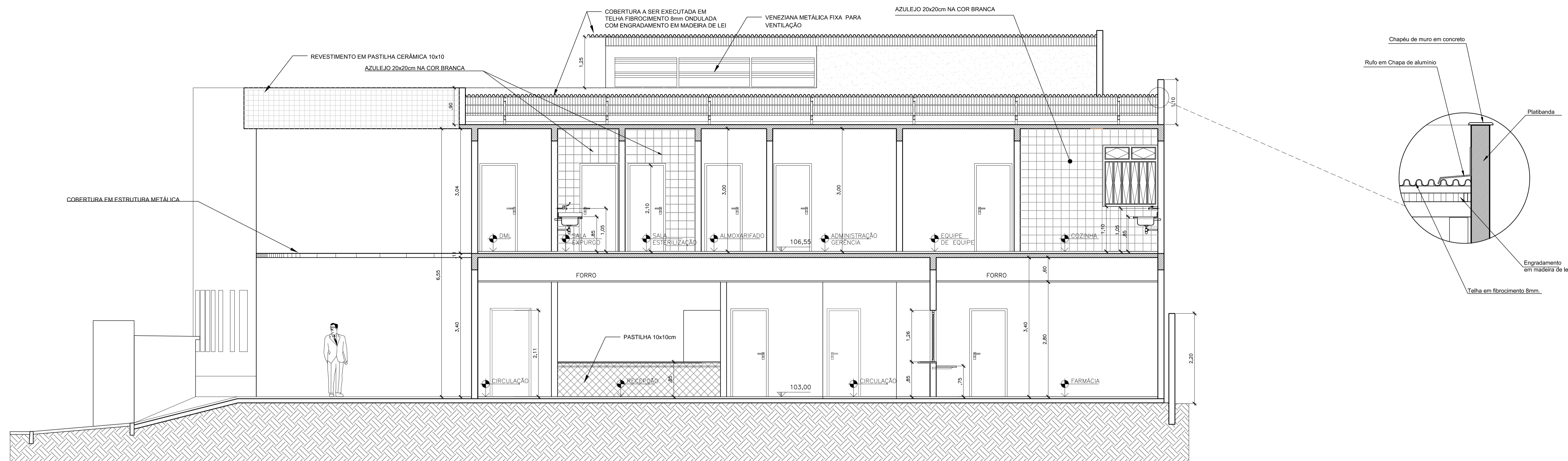
CORTE 3 ESCALA: 1:50
