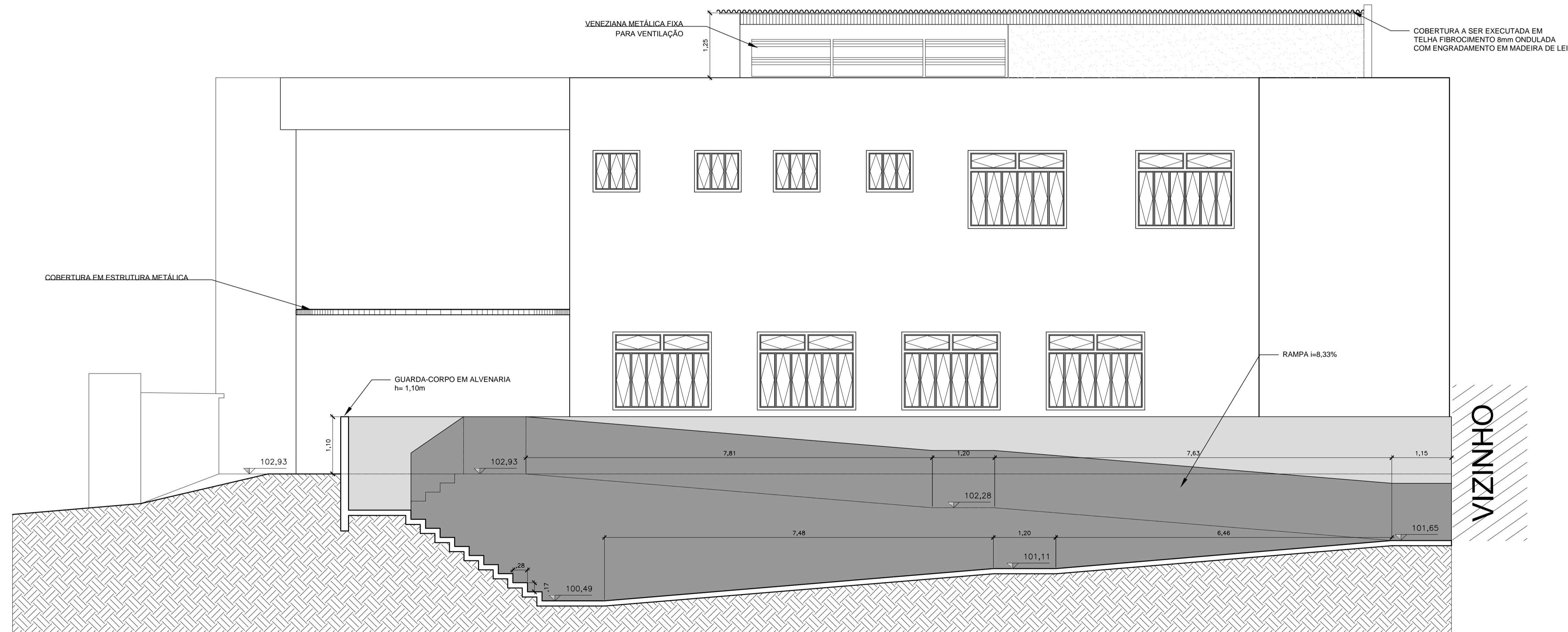
CORTE 4 ESCALA: 1:50
