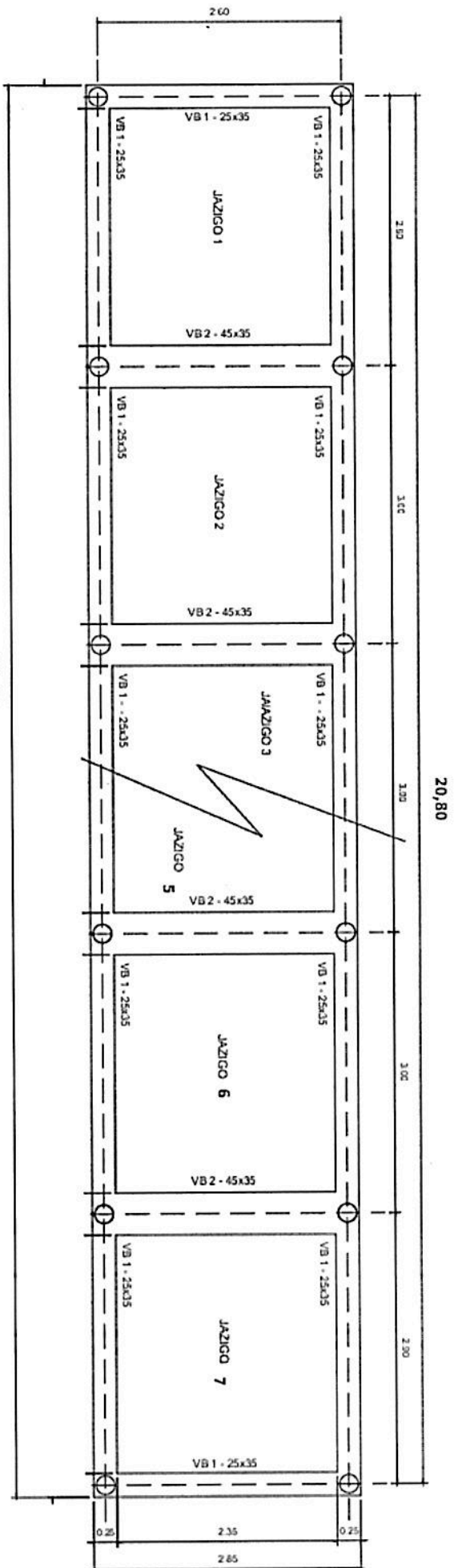
LOCALIZAÇÃO DAS ESTACAS sem escala
