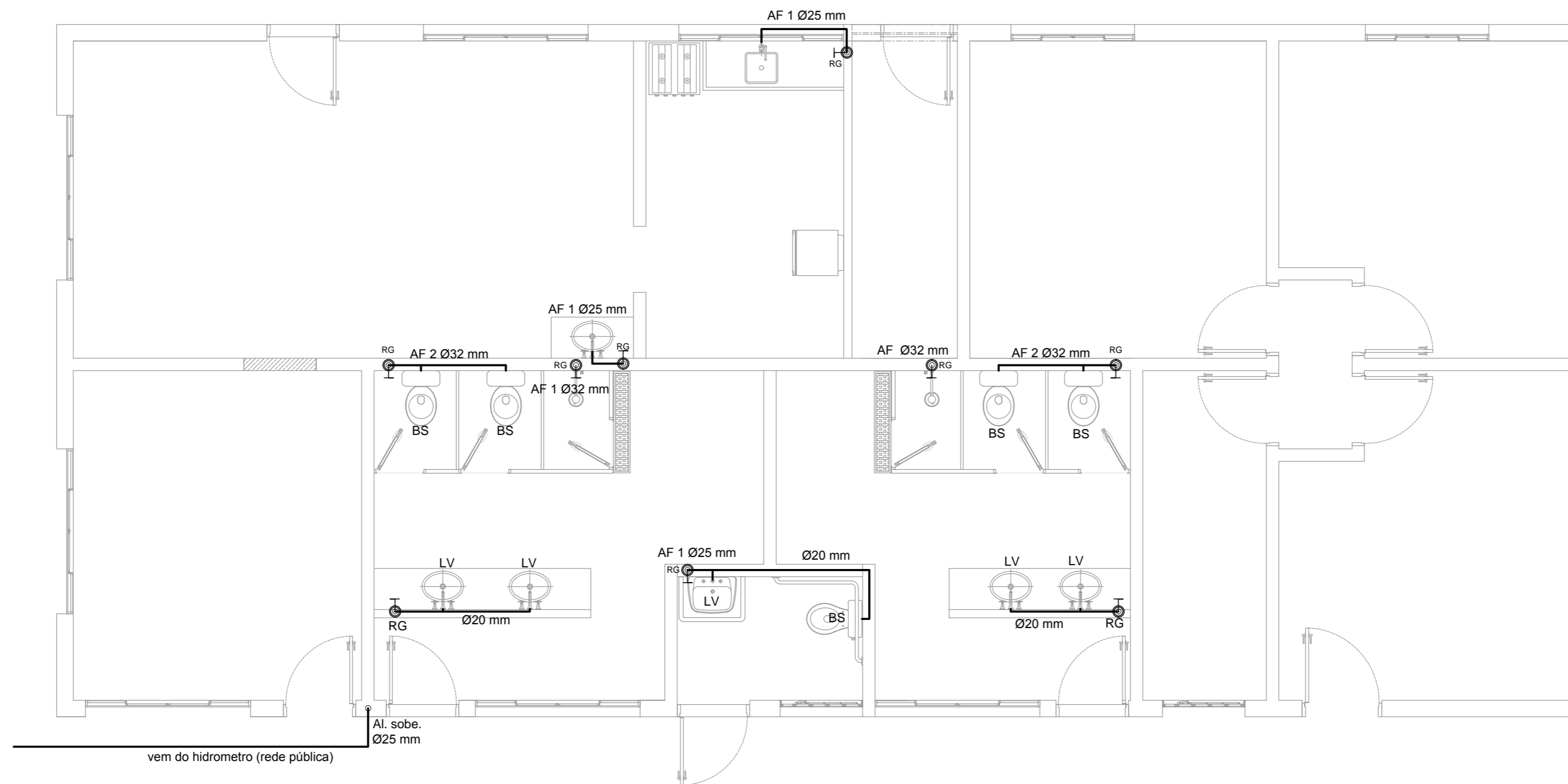
3 PLANTA - ÁGUA FRIA Scl: 1:50
