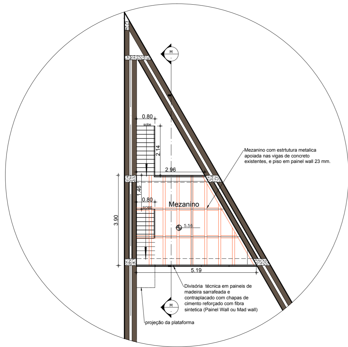
MEZZANINO - NÍVEL 5.56 Scale: 1:100
