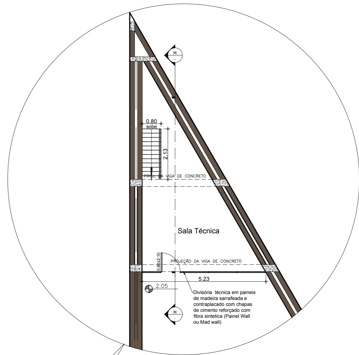
SALA TÉCNICA - NÍVEL 2.05 Scale: 1:100
