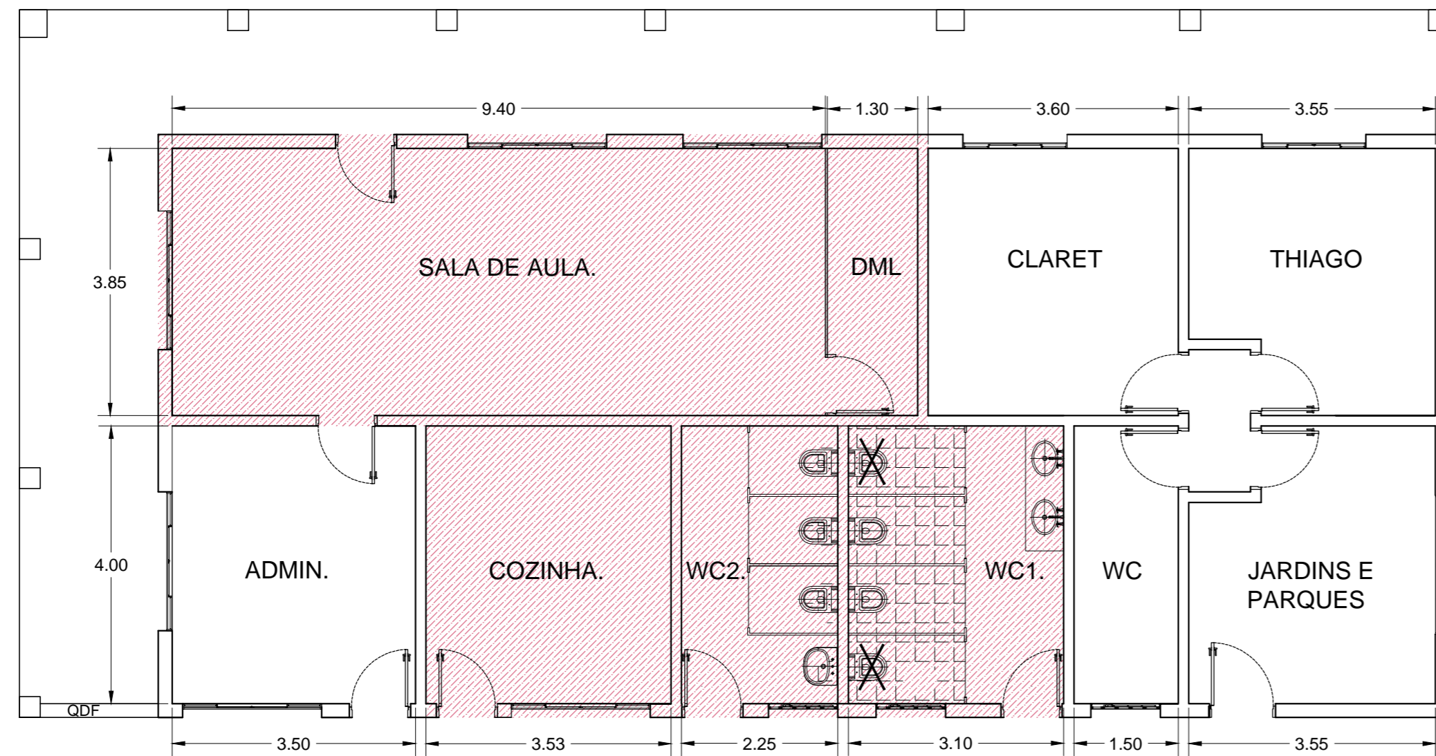
1 PLANTA CADASTRO 2016 Esc: 1:100
