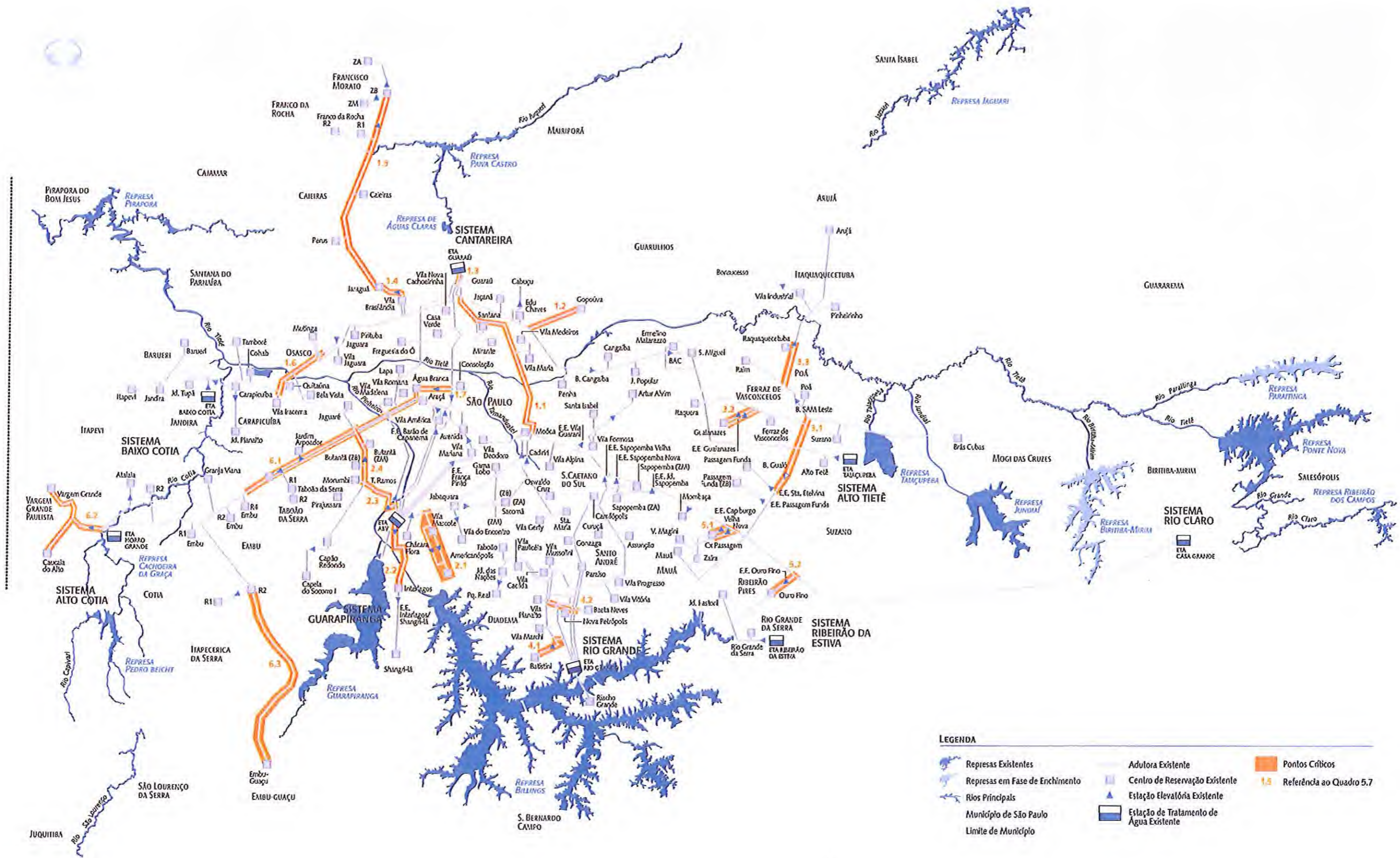
Figura 1.16: Sistema de Abastecimento de Água da RMSP e Pontos Críticos
